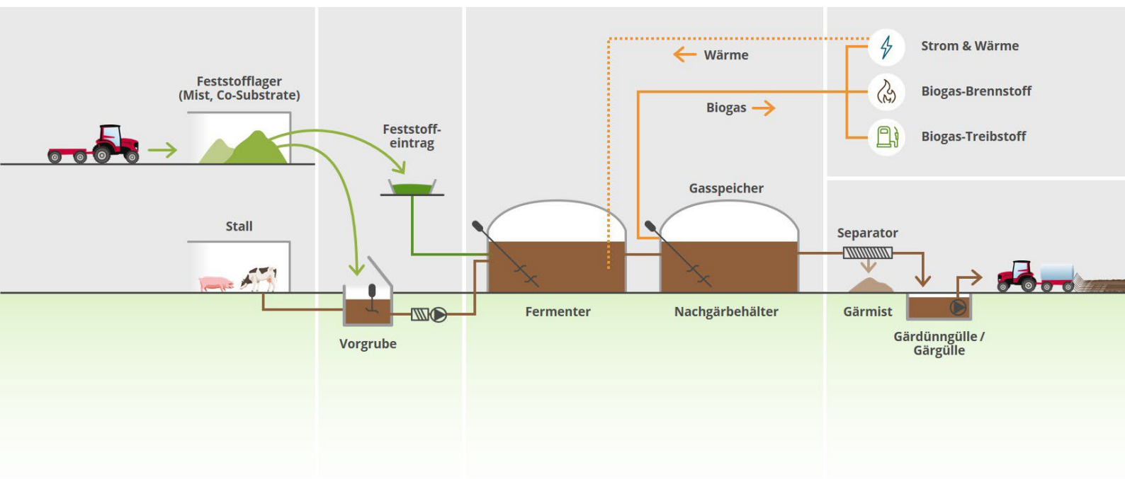
Abbildung 2: Schema einer landwirtschaftlichen Biogasanlage. (Quelle: Ökostrom Schweiz)
