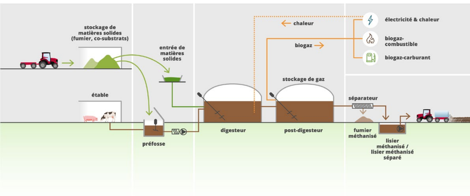
Figure 2: Schéma d'une installation de biogaz agricole. (Source : Ökostrom Schweiz)
